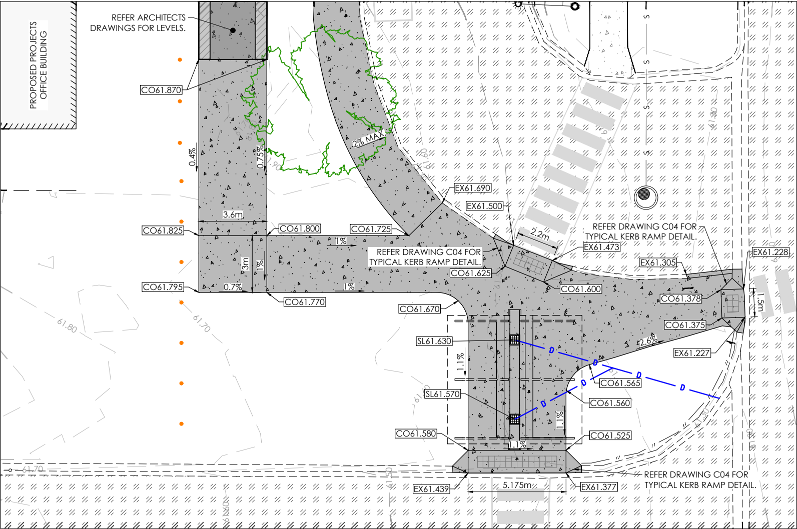
HAT STAND AREA LEVELS
